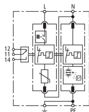
Prinzipschaltbild DG M TT 2P ACI 275 FM
