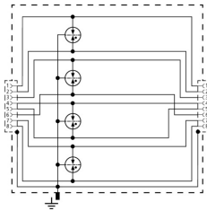
Prinzipialschaltbild DPA M CLD RJ45B 48
