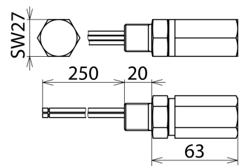
Maßbild DPI CD EXI+D 2X24 N
