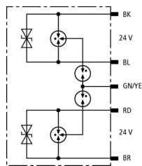
Principalschaltbild DPI CD EXI+D 2X24 N
