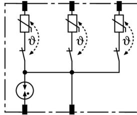
Prinzipschaltbild DR MOD 4P 255 SN1871
